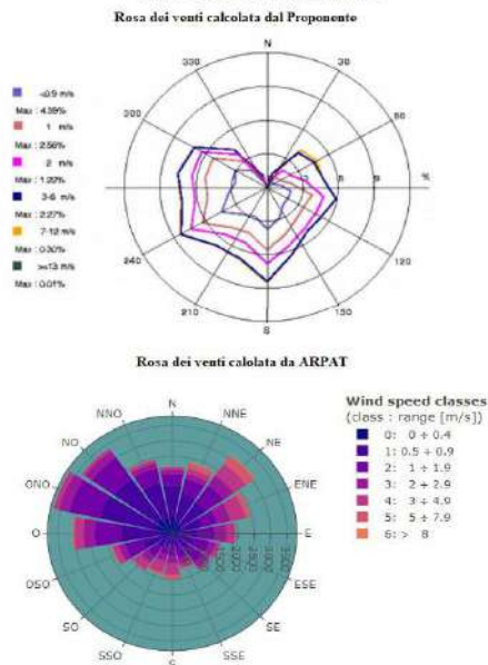
Figura 1: confronto fra le rose dei venti (in alto quella del proponente, in basso quella elaborata da ARPAT utilizzando i dati originali della stazione TOS11000082).
